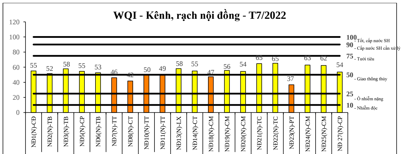
Biểu đồ 3: Diễn biến WQI kênh, rạch nội đồng tháng 7/2022
