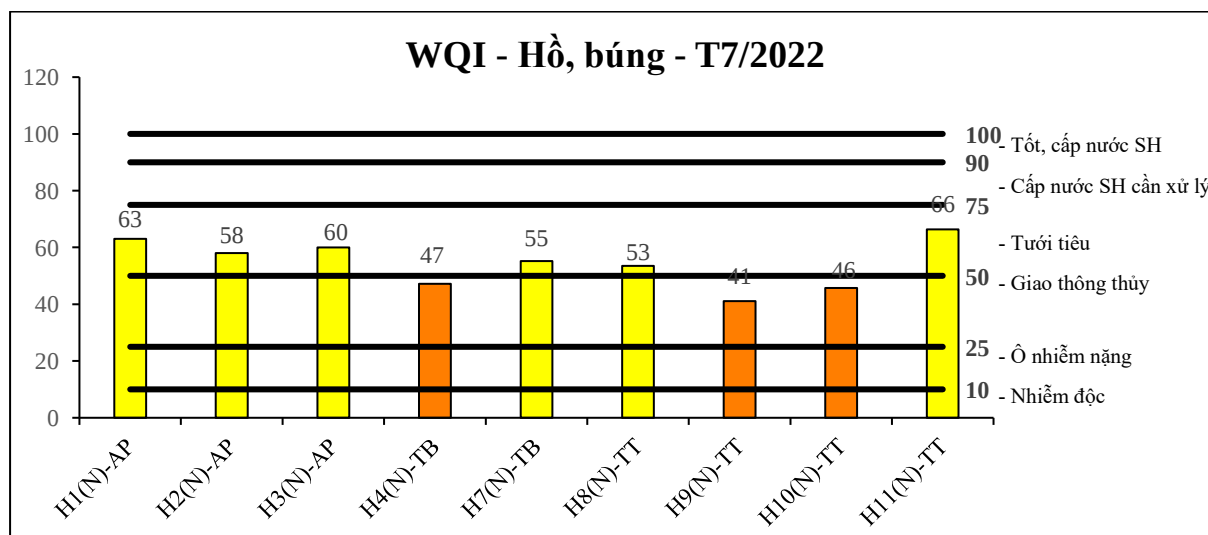
Biểu đồ 4: Diễn biến WQI hồ, búng tháng 7/2022
