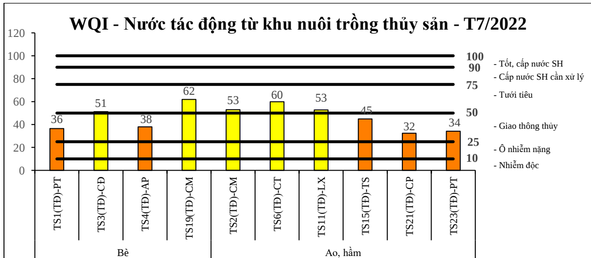
Biểu đồ 9: Diễn biến WQI khu vực nuôi trồng thủy sản tháng 7/2022
