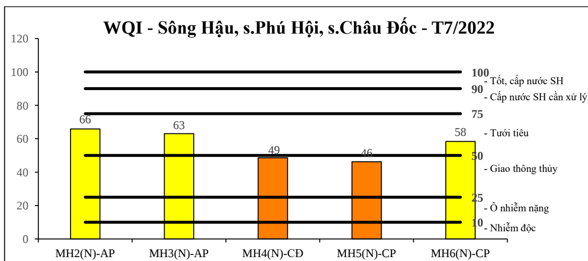
Biểu đồ 2: Diễn biến WQI s.Hậu, s.Phú Hội, s.Châu Đốc tháng 7/2022
