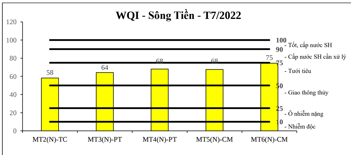
Biểu đồ 1: Diễn biến WQI đầu sông Tiền tháng 7/2022
